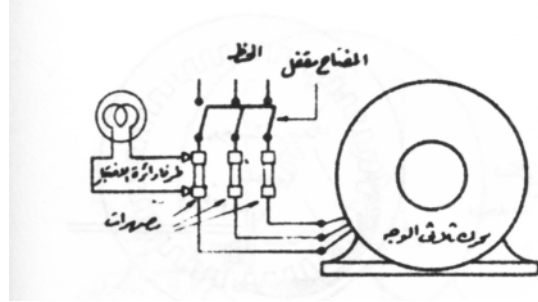
اختبار المصهر وهو في دائرة المحرك (فيوز - fuse)
