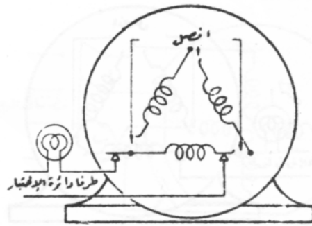
محرك موصل دلتا يتم فحصه بمصباح اختبار
